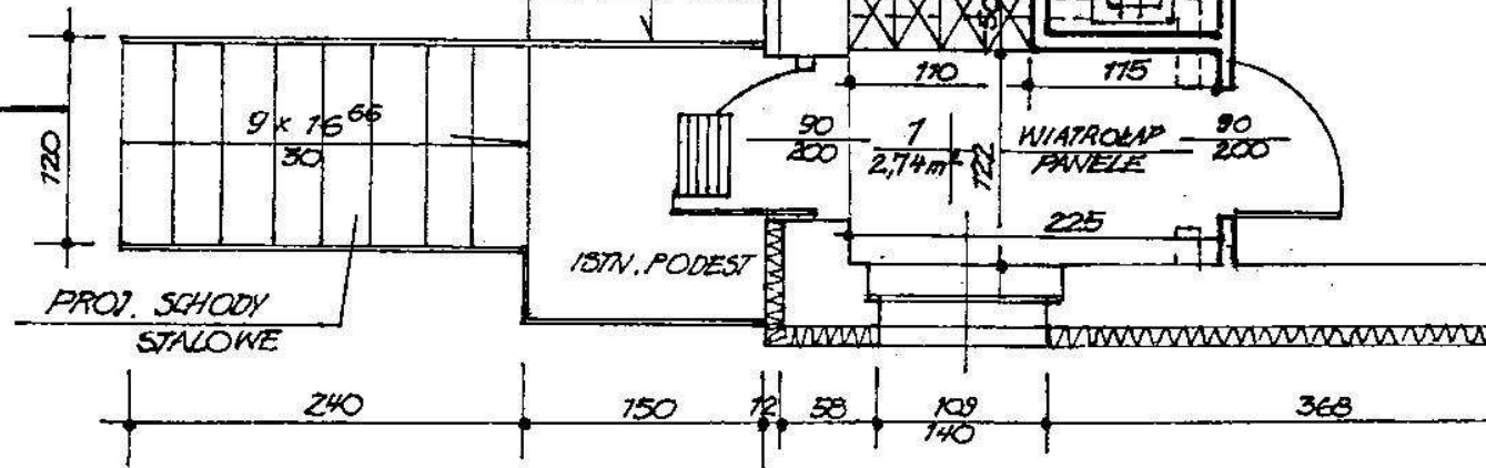
RZUT 1:50
