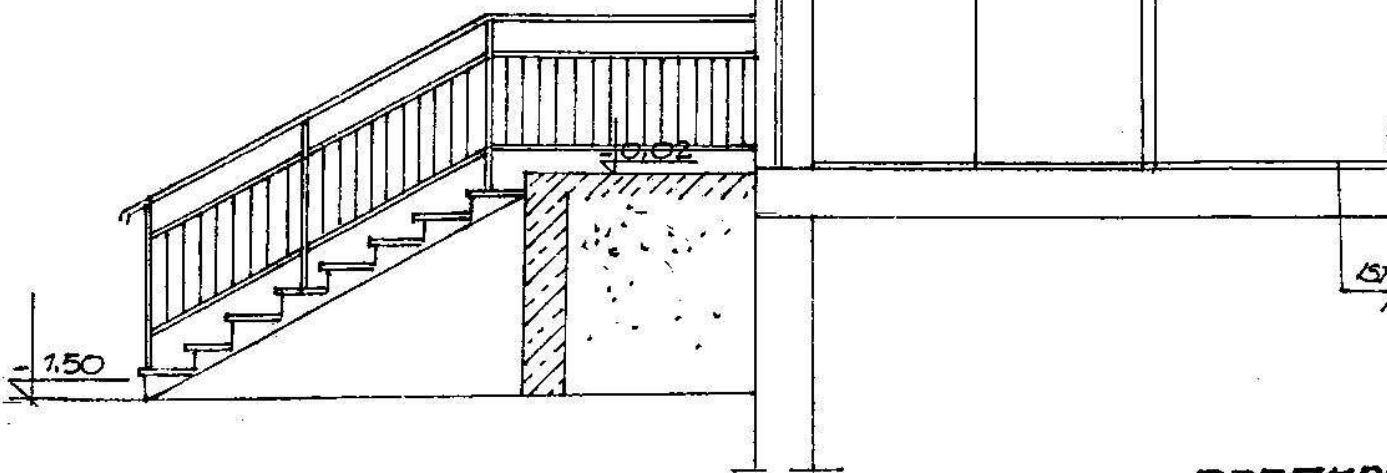
PRZEKROJ 1:50
