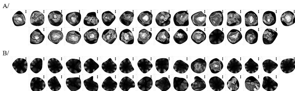
Ryc. 1. Porównanie tomogramów 30 jodeł z rezerwatu Uhryń (A) i z Gorczańskiego PN (B)
